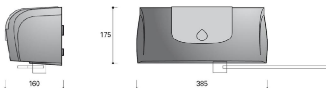
Afmetingen
