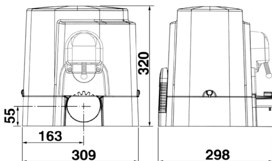
Afmetingen
