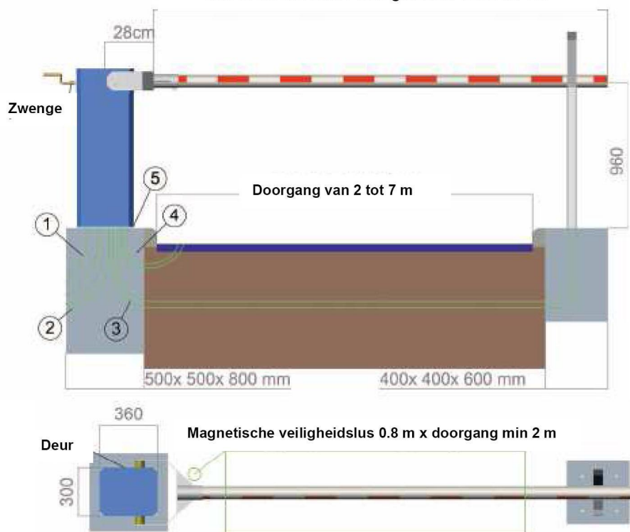
Arm in alu van 2 tot 7 m of glasvezel van 2 tot 4 m
