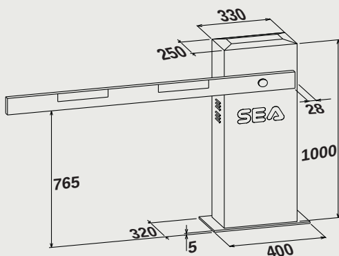
Maße (mm)
