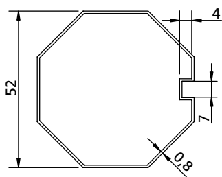
ACHTHOEKIG Ø 52 OCTOGONAL Ø 52
