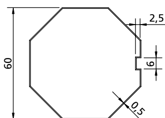
ACHTHOEKIG Ø 60 OCTOGONAL Ø 60
