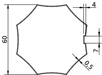
STER Ø 60 ÉTOILE Ø 60
