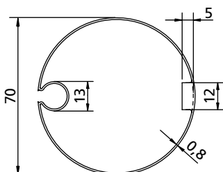
NAAFKAP Ø 70 GORGE Ø 70
