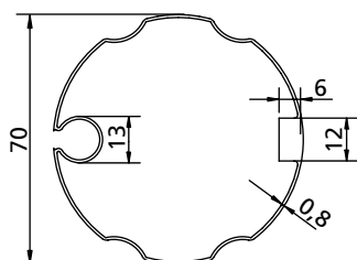
GEGOLFDE NAAFKAP Ø 70 GORGE Ø 70 ONDULÉE
