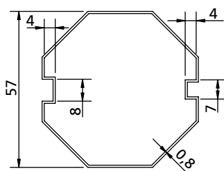
ACHTHOEKIG Ø 57 OCTOGONAL Ø 57
