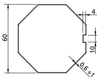
ACHTHOEKIG Ø 60 OCTOGONAL Ø 60
