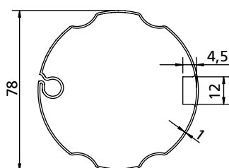
ROLLERBAT NAAFKAP Ø 78 GORGE Ø 78 ROLLERBAT
