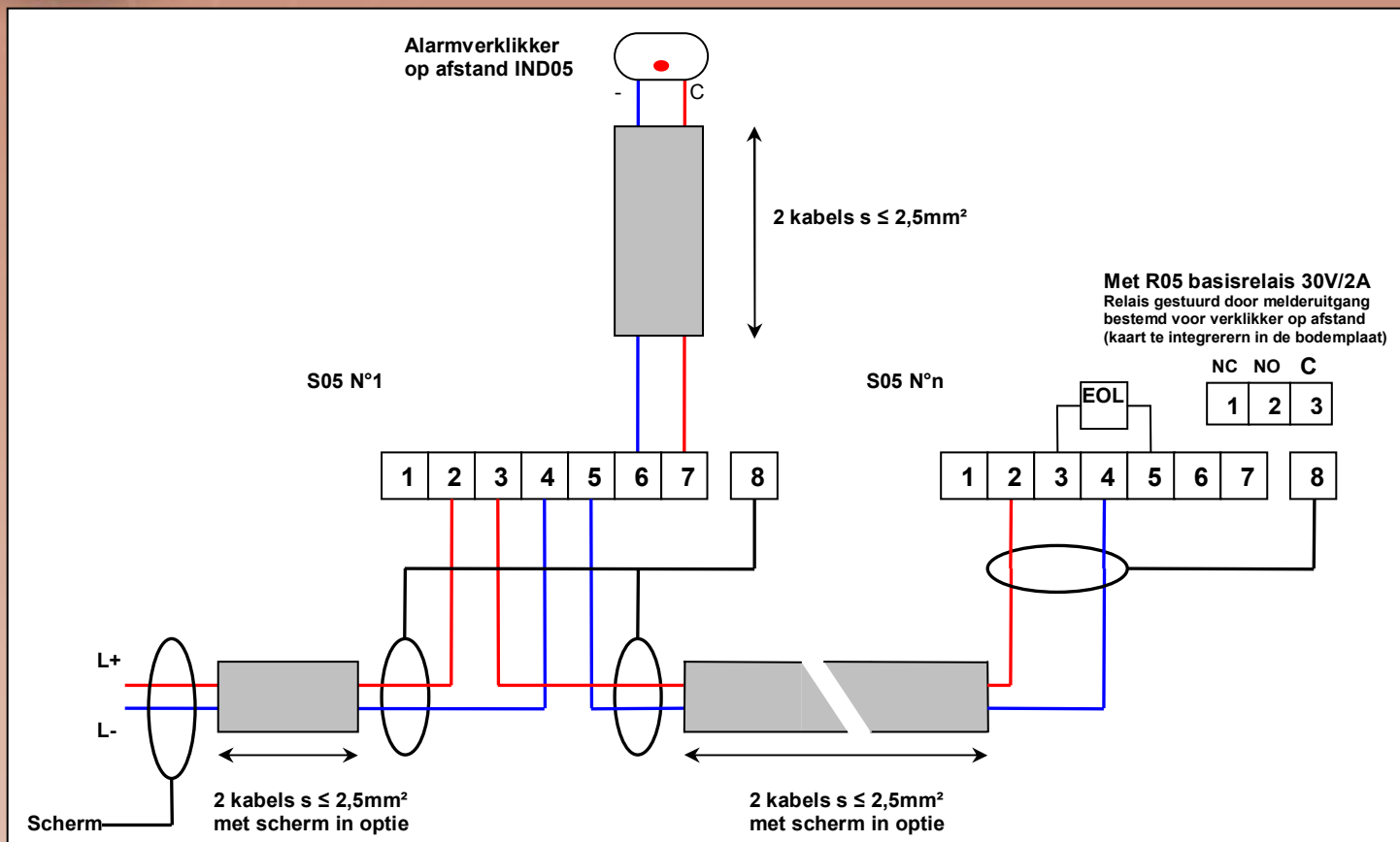
Bodemplaat S05
