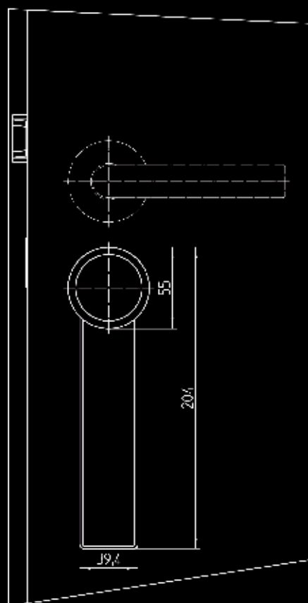
Système de fermeture de portes - Variante avec bouton tournant
