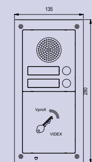
2 push button panel Posto esterno a 2 pulsanti
