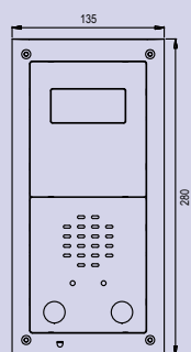
2 push buttons panel Posto esterno a 2 pulsanti
