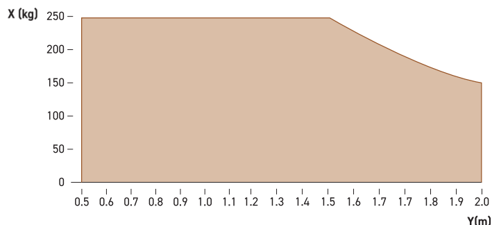
Grafiek 1 - Gebruikslimieten
