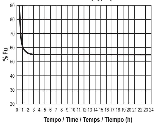
TOP291E(R)(/S)
