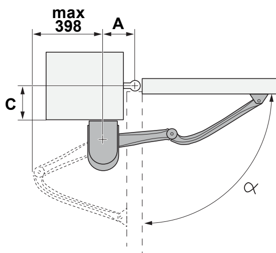
Exemple d'installation 162271
