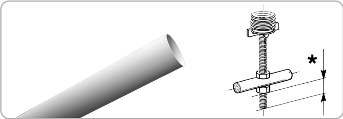
Asta 6 mt. Ø 100 mm spessore 2 mm senza mozzo L = 6 mt. N.B.: Al momento dell'ordine richiedere le molle di bilanciamento apposite (n° 1 mm 5,5 e n° 1 mm 6). cod. ACG8497
