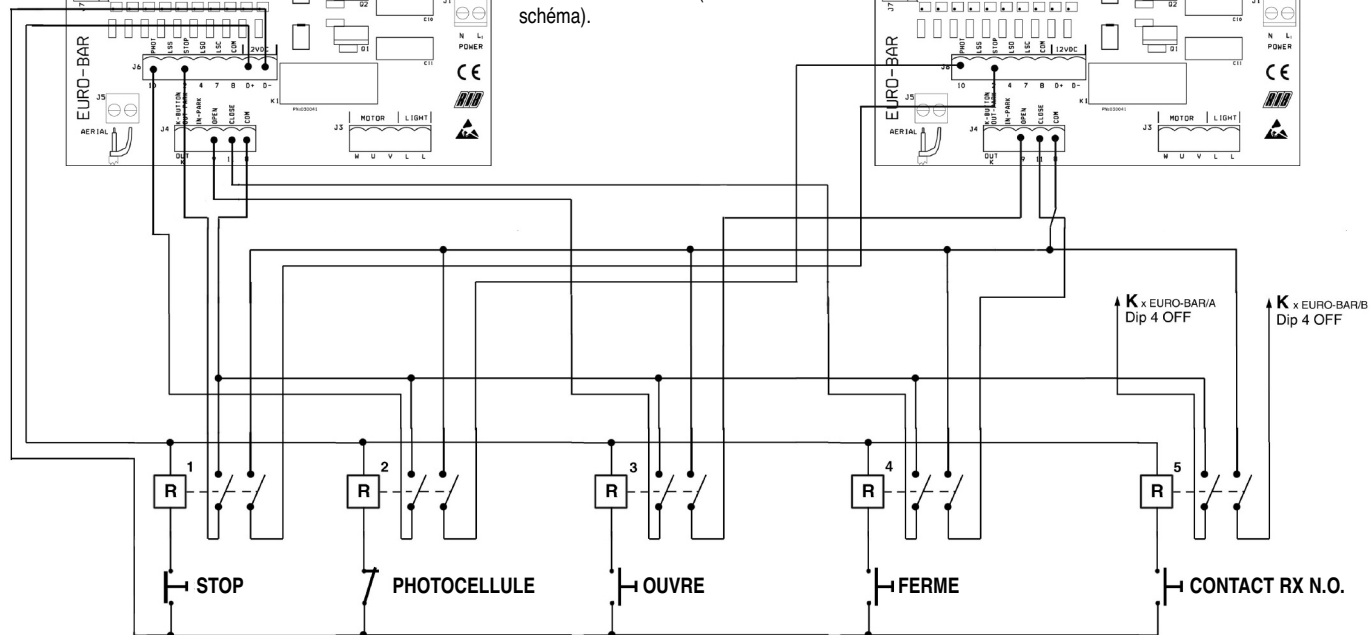
RELAIS 12Vdc POUR 5 CONTACTS DOUBLES
