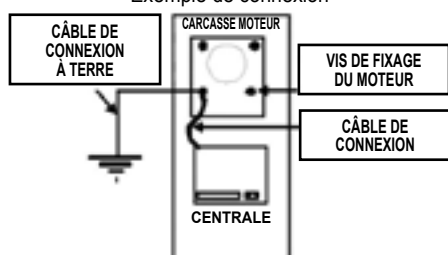
Exemple de connexion
