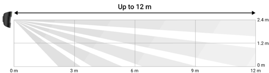
Angle de vue vertical du détecteur
