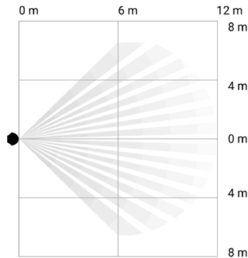
Angle de vue horizontal du détecteur
