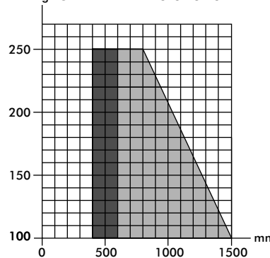
Kg GRAFIEK NEPTIS-SL en SM
