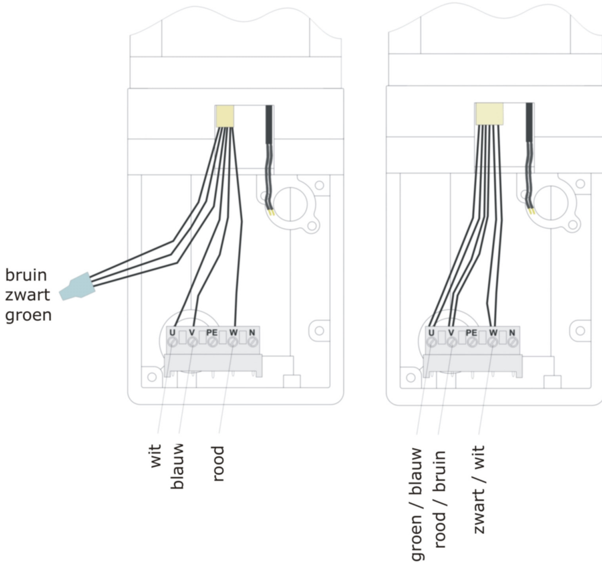
3x400 V
