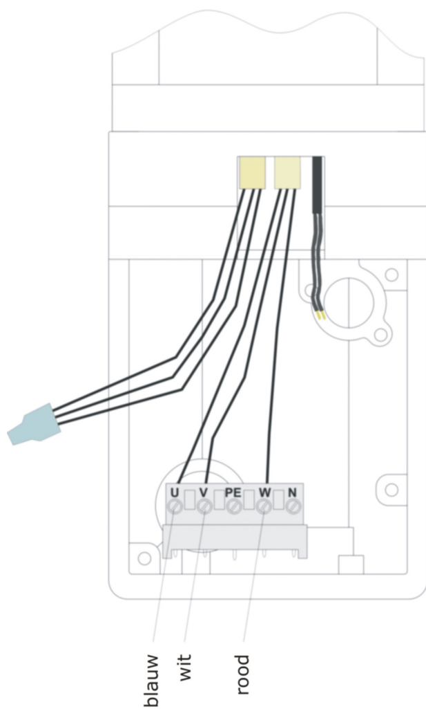
3x400 V
