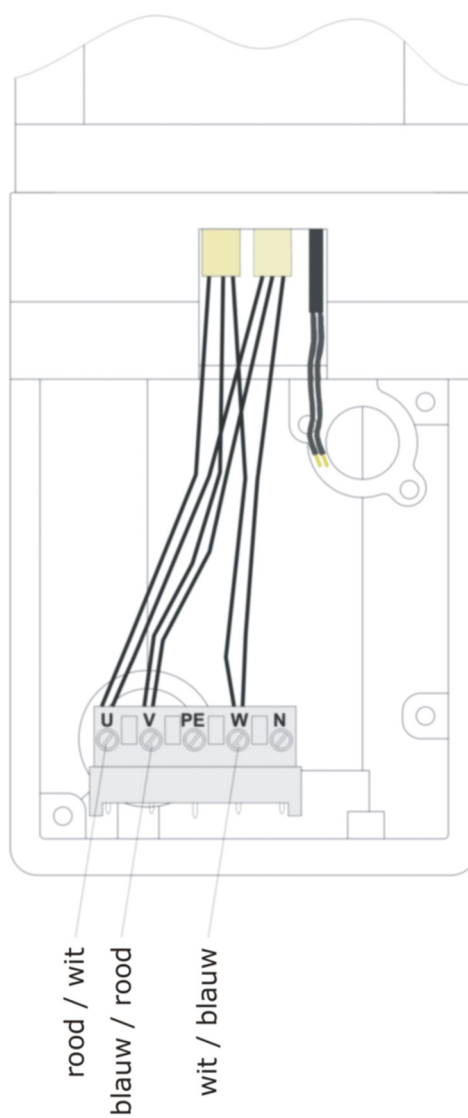
3x230 V
