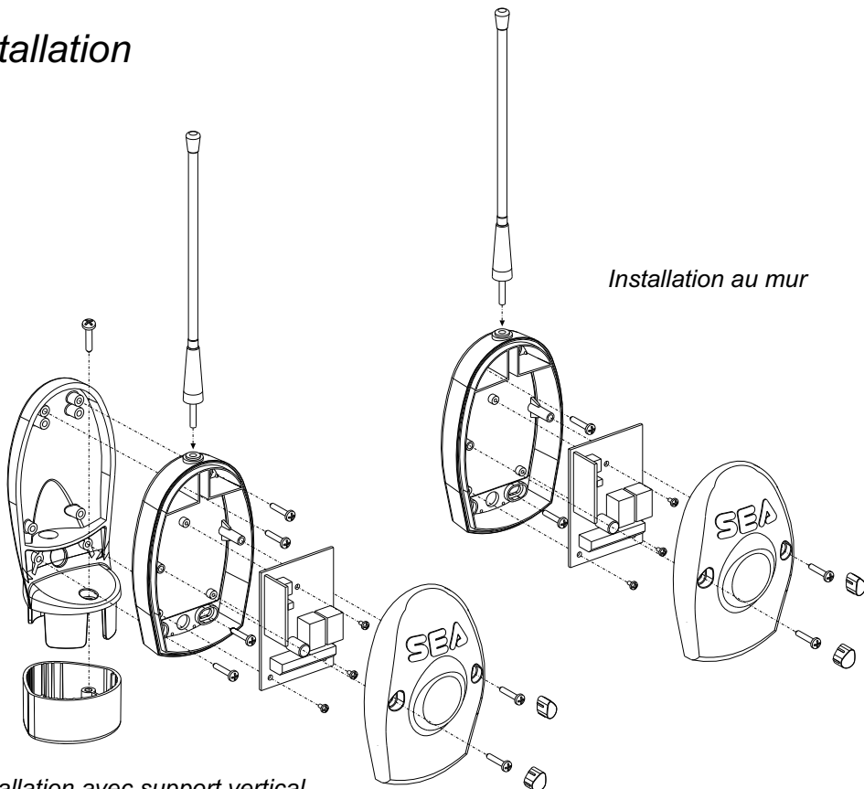
Installation avec support vertical
