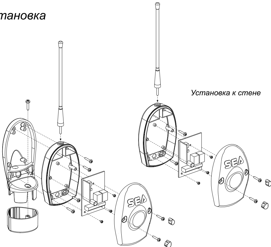
Установка с вертикальной опорой
