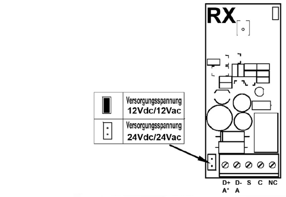
Rückseite der RX-Platine, Seite Schweißnähte Konfigurierung des anzuwendenden Kontaktes.
