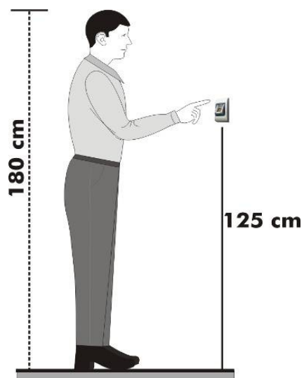
Montagepositie
