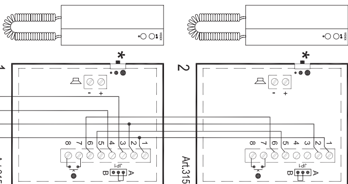
Posizione ponticello mobile JP1 Jumper JP1 position
