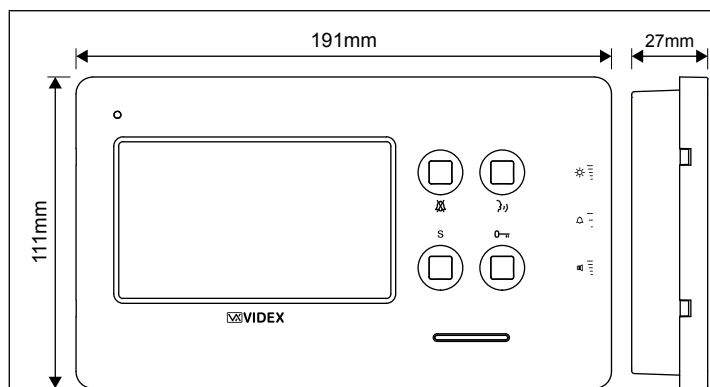
Fig. 1 Partie avant
