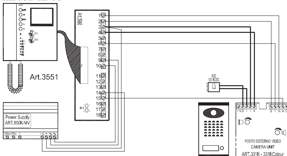
VIDEOCITOFONO / VIDEOPHONE
